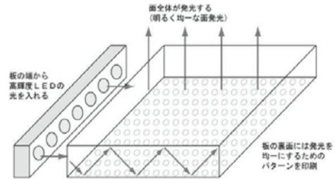
光拡散板(導光板)の仕組み
